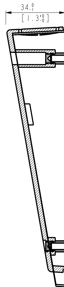
section A-A
